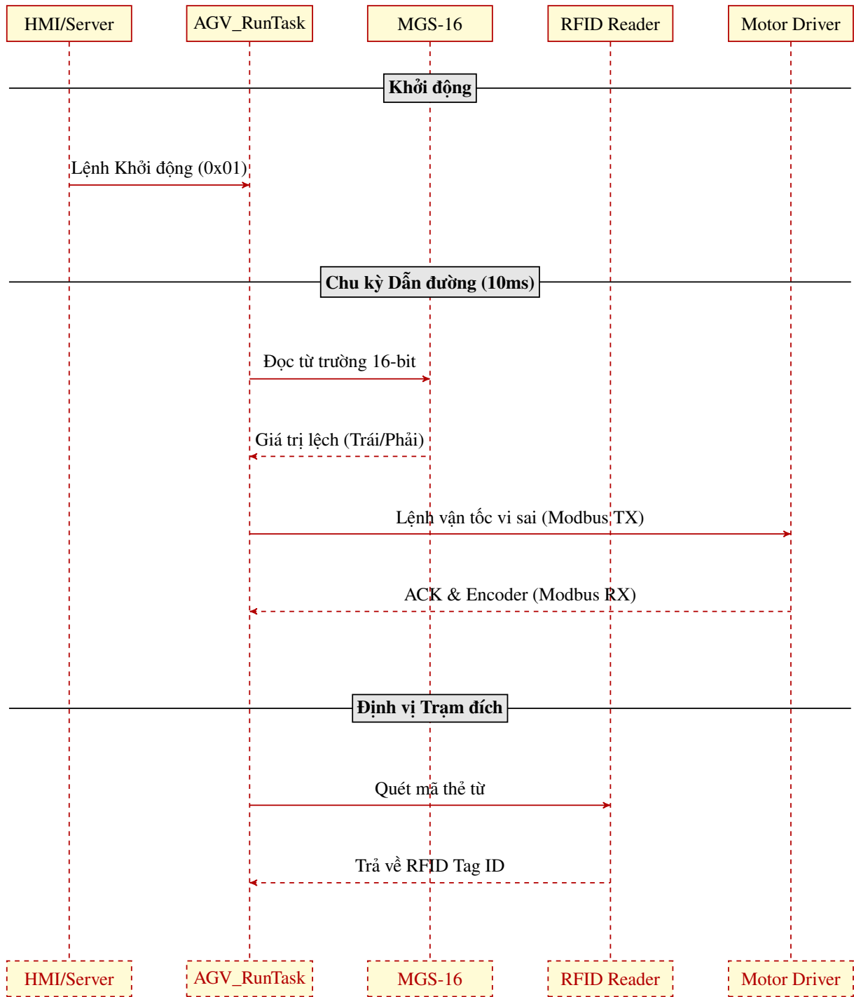
Hình 4.8 Sơ đồ tuần tự quá trình dẫn đường và nhận dạng trạm RFID.
