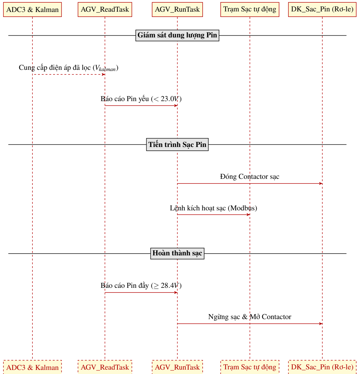
Hình 4.11 Sơ đồ tuần tự quá trình giám sát Pin và sạc tự động.
