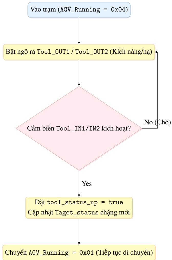
Hình 4.5 Sơ đồ tuần tự quy trình nâng/hạ móc kéo hàng tự động.
