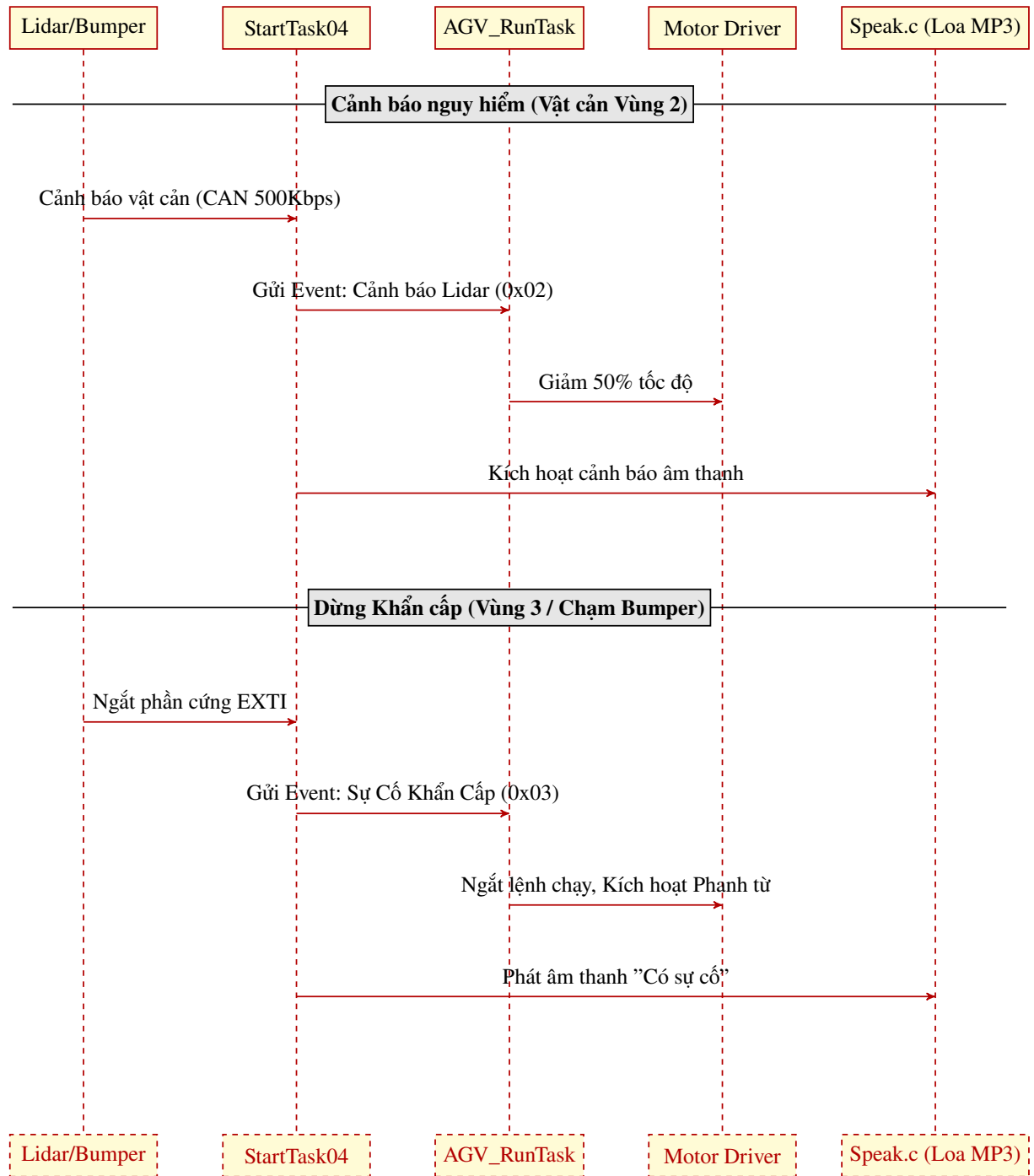
Hình 4.9 Sơ đồ tuần tự luồng giám sát an toàn và xử lý sự cố khẩn cấp.
