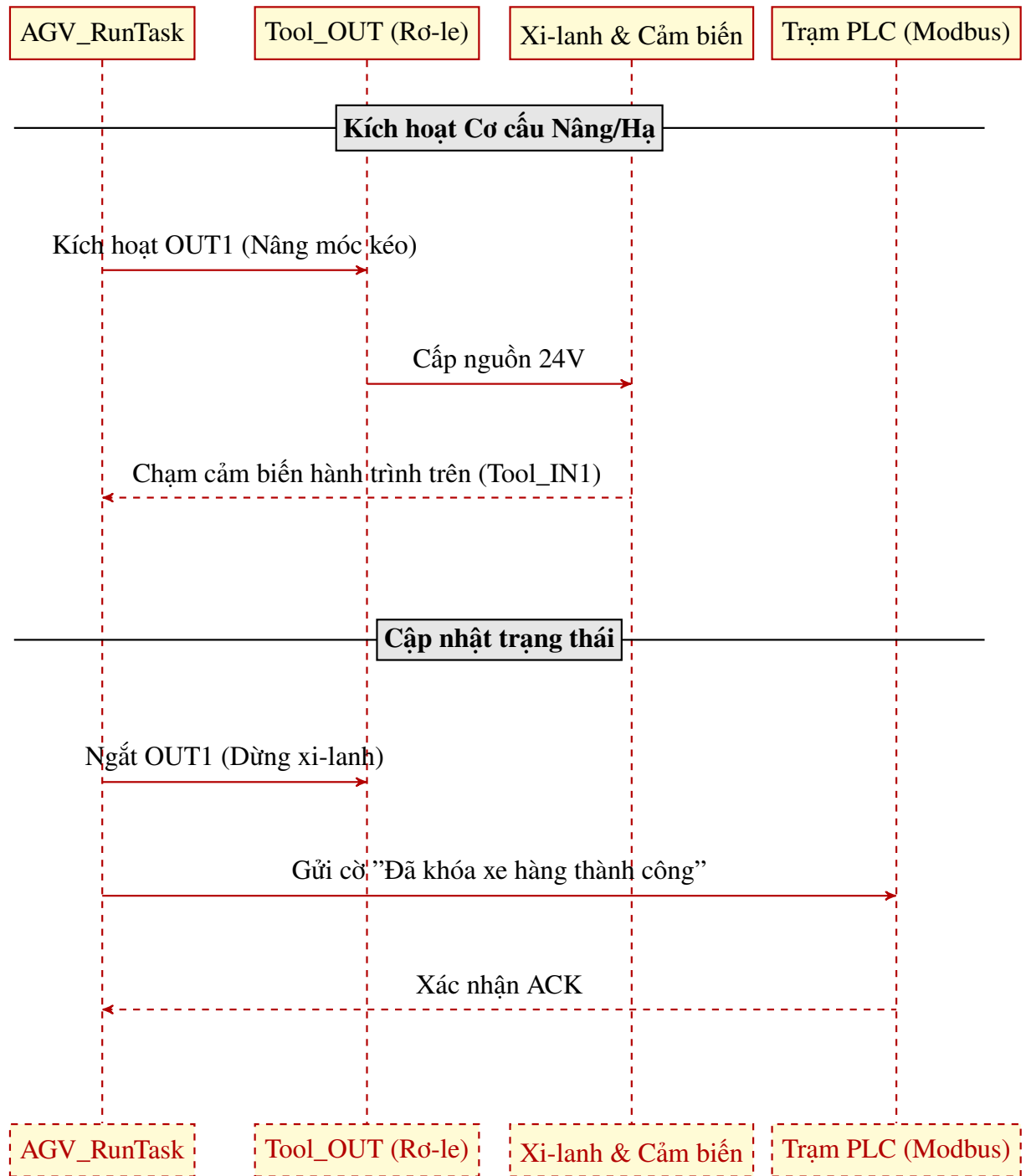
Hình 4.10 Sơ đồ tuần tự hoạt động của cơ cấu móc kéo xe hàng.
