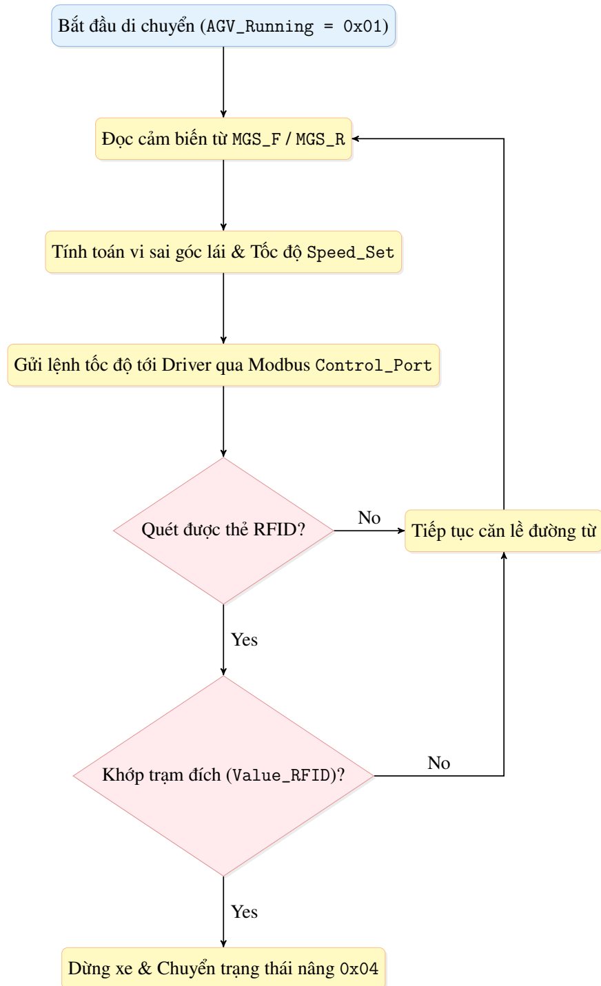
Hình 4.3 Sơ đồ thuật toán dẫn đường từ và định vị vị trí trạm bằng thẻ RFID.
