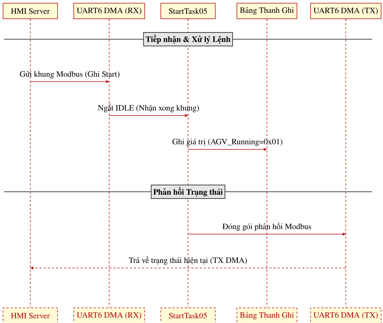
Hình 4.12 Sơ đồ tuần tự giao thức truyền thông Modbus RTU.
